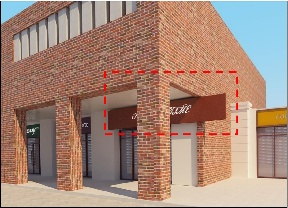
牌匾标识外沿不得超出出挑结构外墙面
